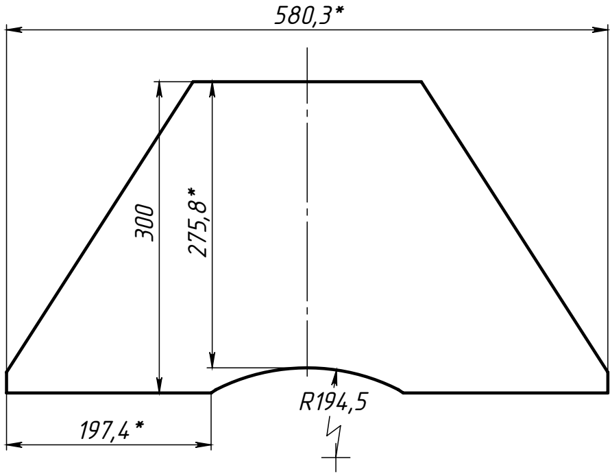
Поз.1 (Корпус) развертка
